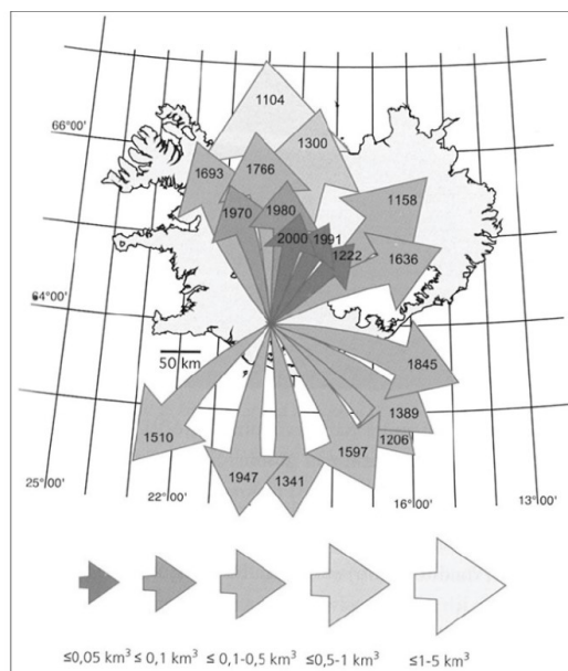
Илл. 2. Густота, направление и дальность выброса тефры (по: Larsen et al. 2013)
