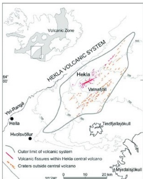
Илл. 1. Вулканическая система Гекла (по: Larsen et al. 2013)
